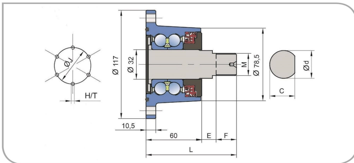
Размеры (мм) Dimensions (mm)
